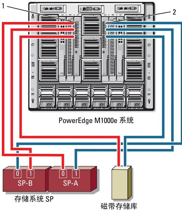
图 2-7. 存储系统和磁带存储库的布线
